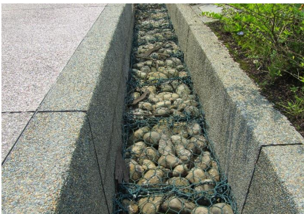
校區週邊水溝運用礫石蛇籠工法
